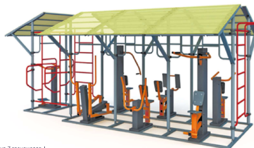
ТРК-1.13 Тренажерная беседка на 4 тренажера | 4,0 * 7,0 * 2,8 м
