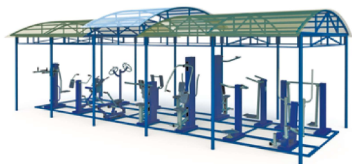
ТРК-1.3 Тренажерная беседка на 14 тренажеров | 10,0 * 4,0 * 3,2 м, площадь 40 м²
