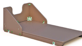
ТРК-1.6 Одиночный окоп | 2,0 * 1,0 * 0,6 м
